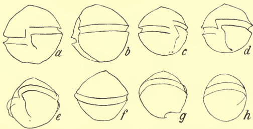
Fig. 27. Glenodinium danicum Pauls. a—b : Ein Exemplar, c—h : ein anderes. a, c, d, e : Verschiedene Ventralansichten. b, h : Linke und rechte Seitenansicht. f, g : Dorsalansichten.
